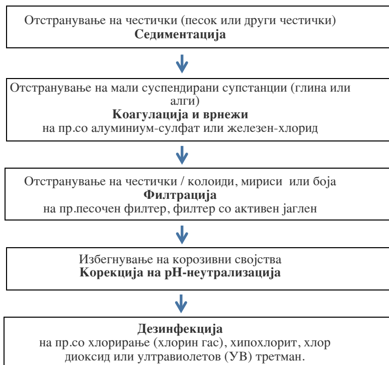
Табела 1: Шема на едноставен систем за третман за површинските води
